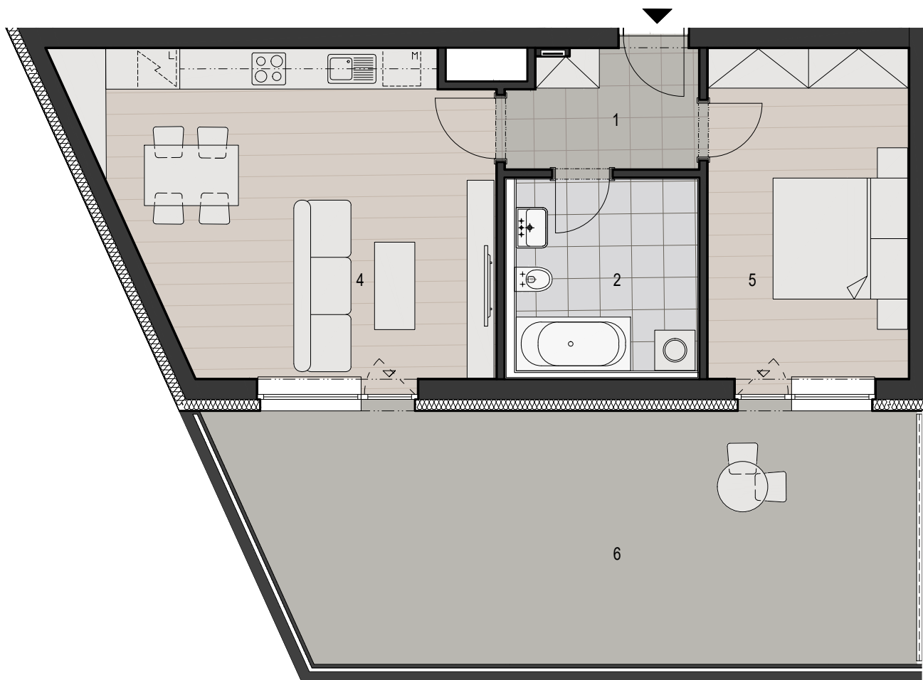
SCHEMA PODLAŽÍ
