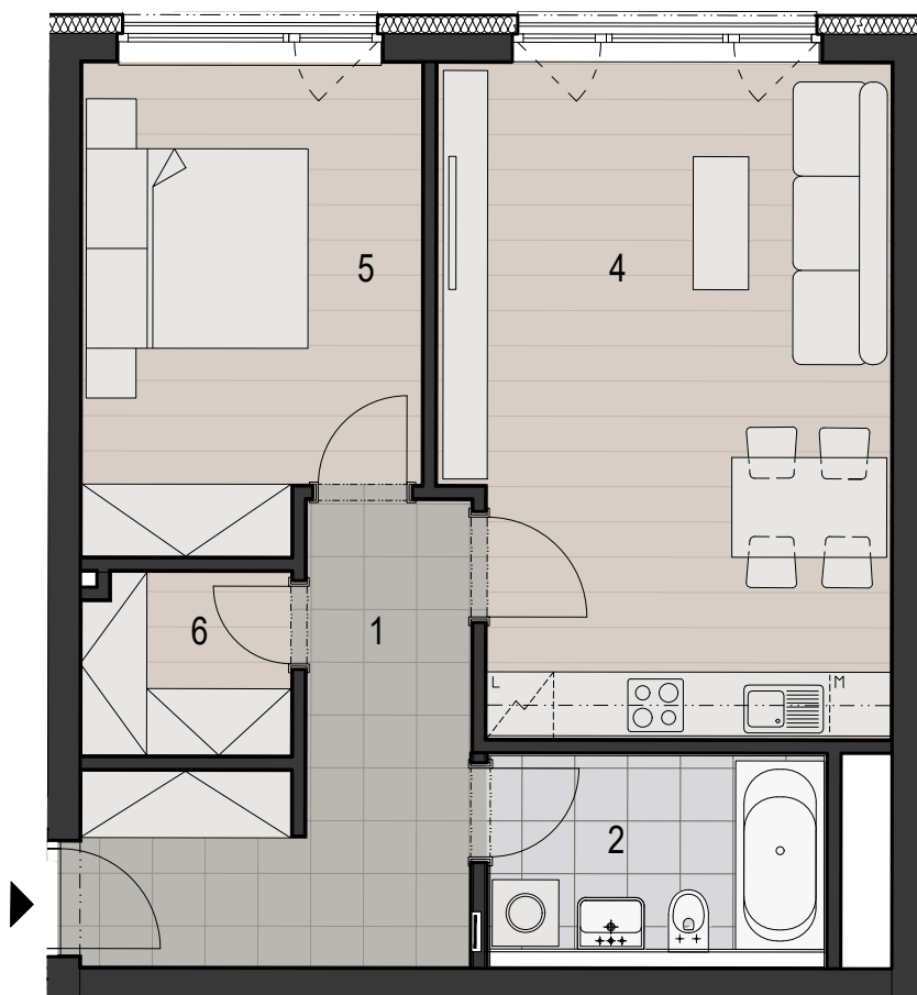
SCHEMA PODLAŽÍ
