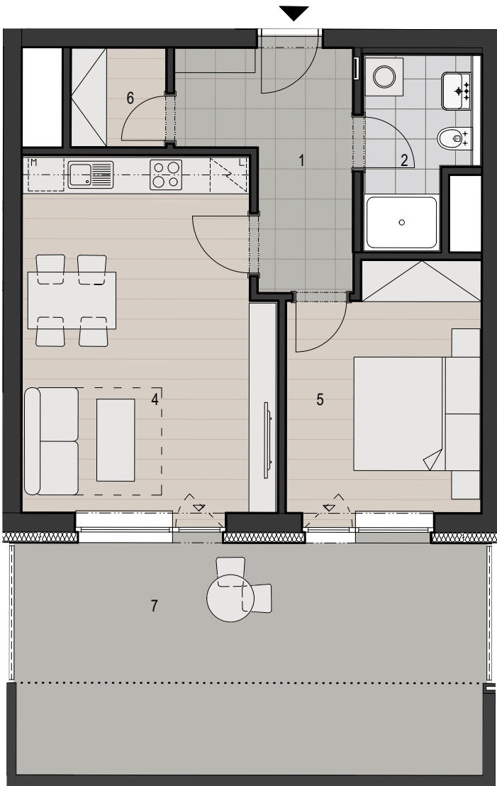
SCHEMA PODLAŽÍ
