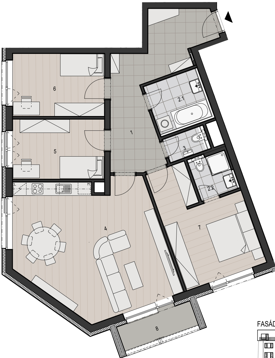
SCHEMA PODLAŽÍ
