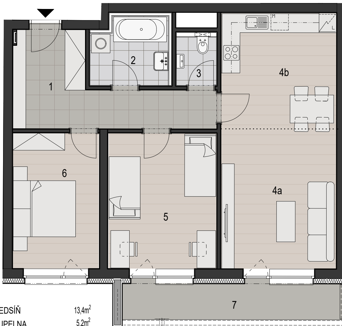
SCHEMA PODLAŽÍ
