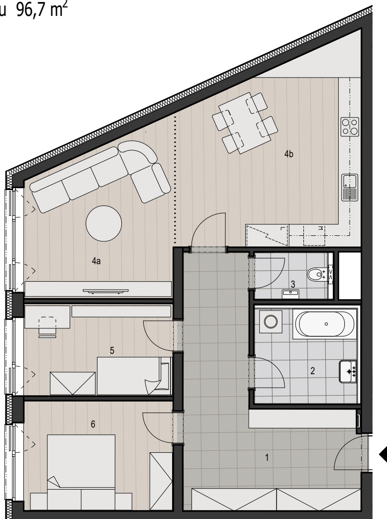
SCHEMA PODLAŽÍ
