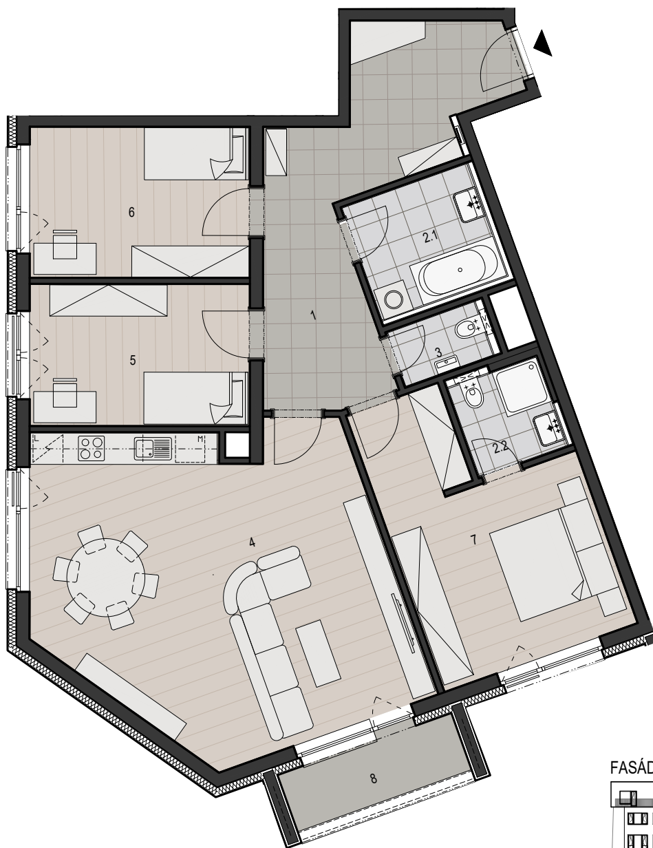
SCHEMA PODLAŽÍ
