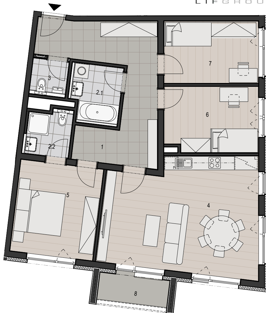
SCHEMA PODLAŽÍ
