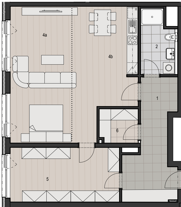
SCHEMA PODLAŽÍ
